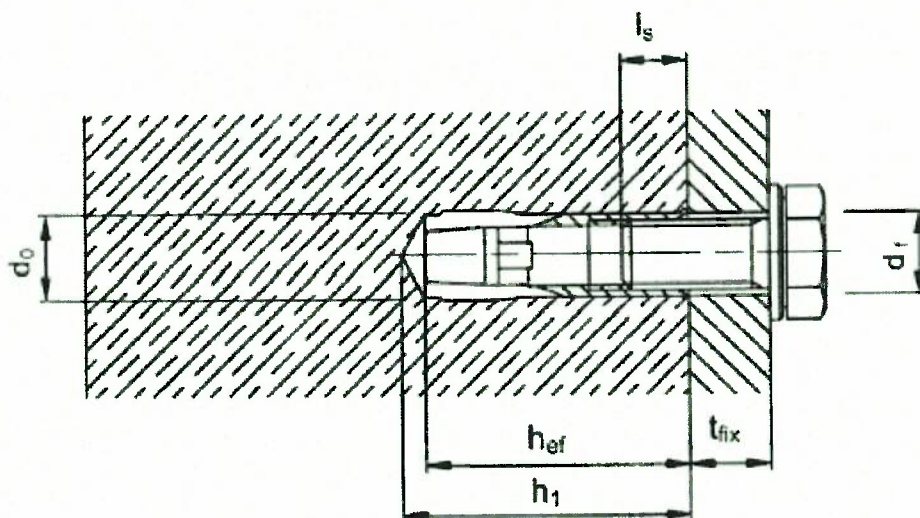
Rys. B1. Parametry montażu tulei kotwiących Hilti HKV
