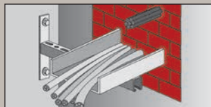
Zaprawa ogniochronna CP 636 / CFS-M RG
